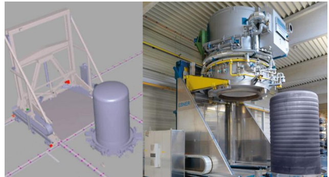
Autonomes Chargiersystem für Haubenöfen
